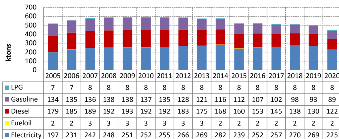
Διάγραμμα 3.40. ΝΣΔΑΕ σενάριο – Προβολή εκπομπών CO 2 τελικής χρήσης ανά ενεργειακό φορέα
