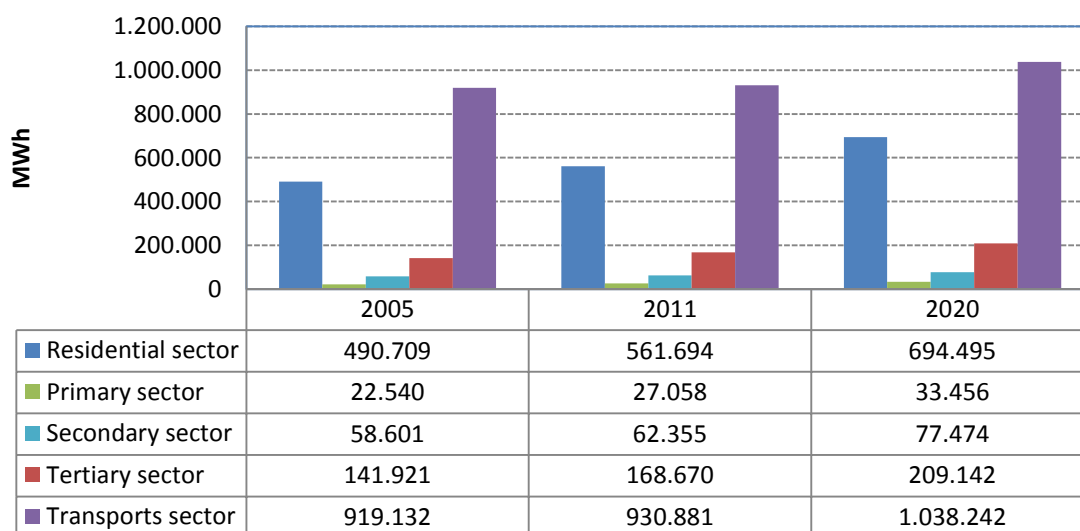
Διάγραμμα 3.21. BAU σενάριο – Τελική ζήτηση ενέργειας ανά κατηγορία δραστηριότητας
