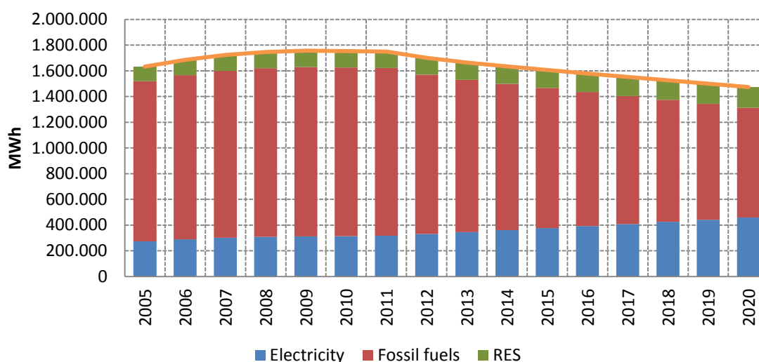
Διάγραμμα 3.32. ΝΣΔΑΕ σενάριο – Τελική ζήτηση ενέργειας ανά ενεργειακή πηγή
