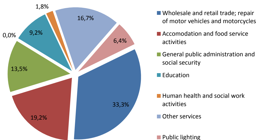
Διάγραμμα 3.16. Εκπομπές CO 2 από τελική χρήση στον τριτογενή τομέα
