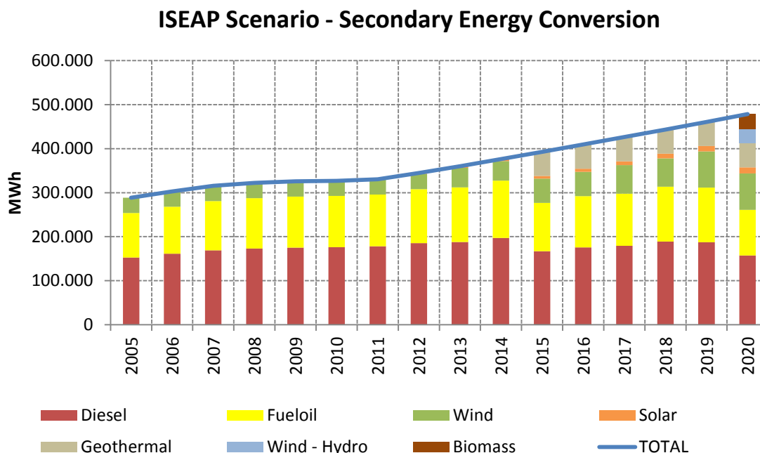
Διάγραμμα 3.36. ΝΣΔΑΕ σενάριο – Προβολή δευτερογενούς μετατροπής ενέργειας έως το 2020
