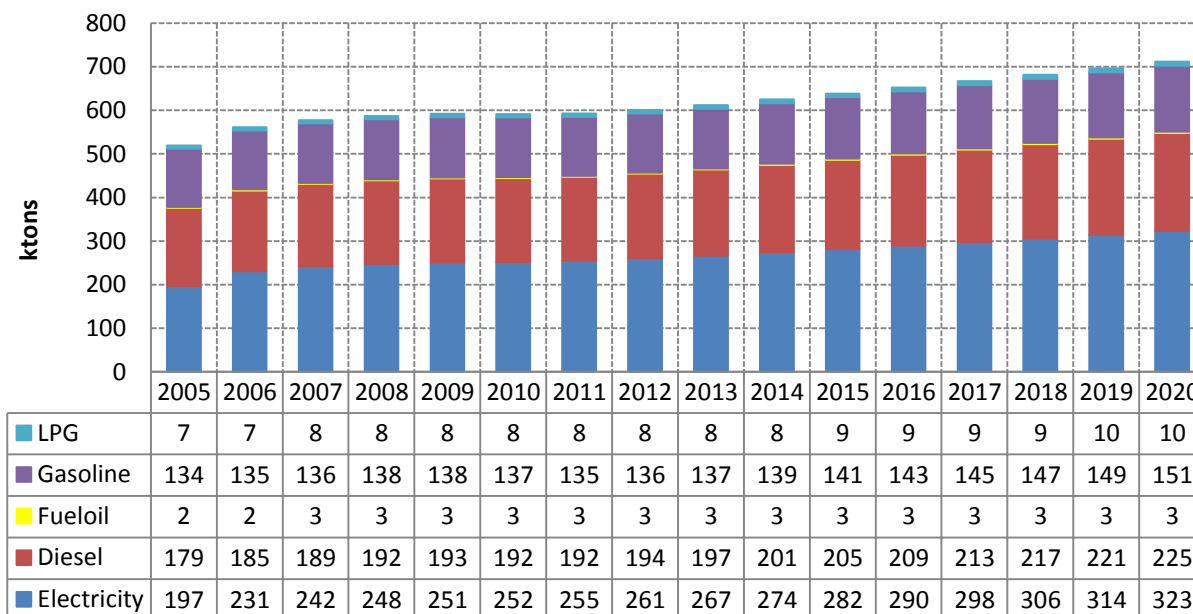
Διάγραμμα 3.27. BAU σενάριο – Προβολή εκπομπών CO 2 τελικής χρήσης ανά ενεργειακό φορέα
