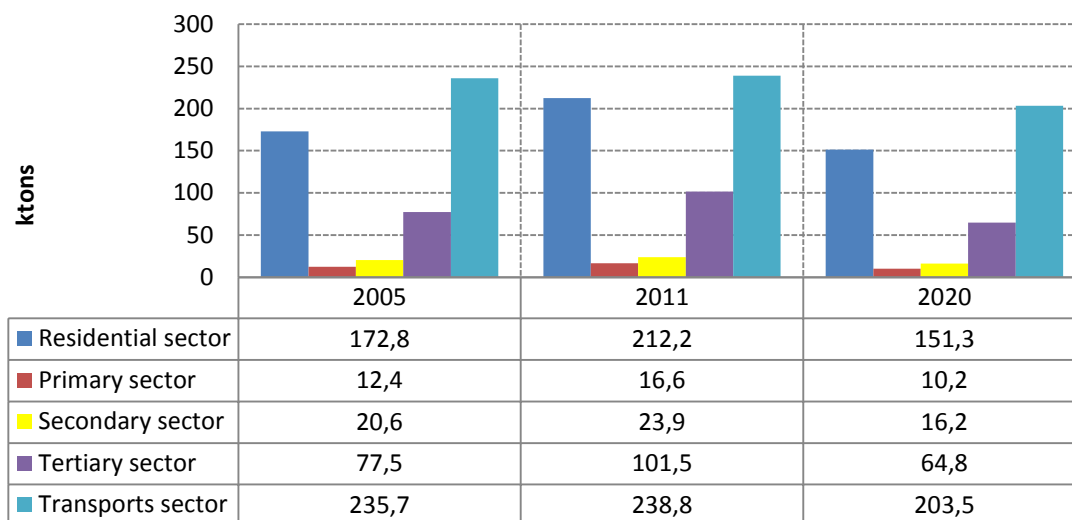
Διάγραμμα 3.42. ΝΣΔΑΕ σενάριο – Προβολή εκπομπών CO 2 τελικής χρήσης ανά ενεργειακό φορέα
