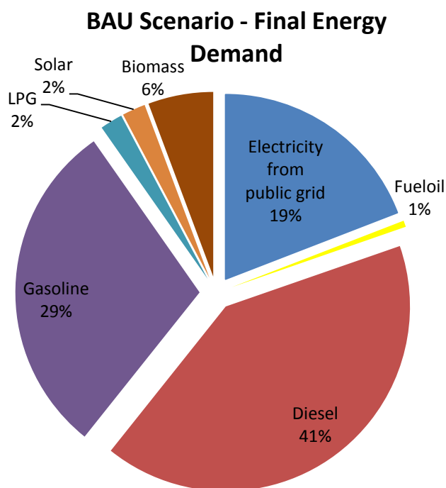
Διάγραμμα 3.22. BAU σενάριο – Τελική ζήτηση ενέργειας ανά ενεργειακό φορέα το 2020
