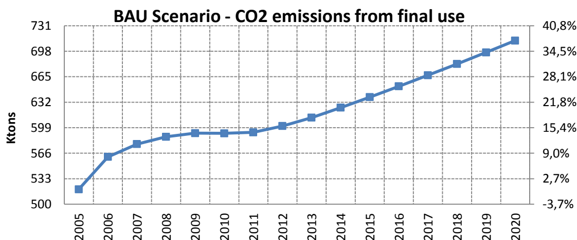
Διάγραμμα 3.19. BAU σενάριο – Προβολή εκπομπών CO 2 από τελική χρήση
