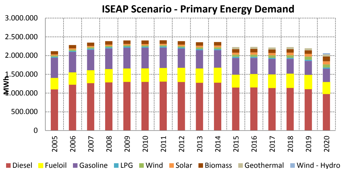
Διάγραμμα 3.38. ΝΣΔΑΕ σενάριο – Προβολή πρωτογενούς ζήτησης ενέργειας ανά ενεργειακό φορέα
