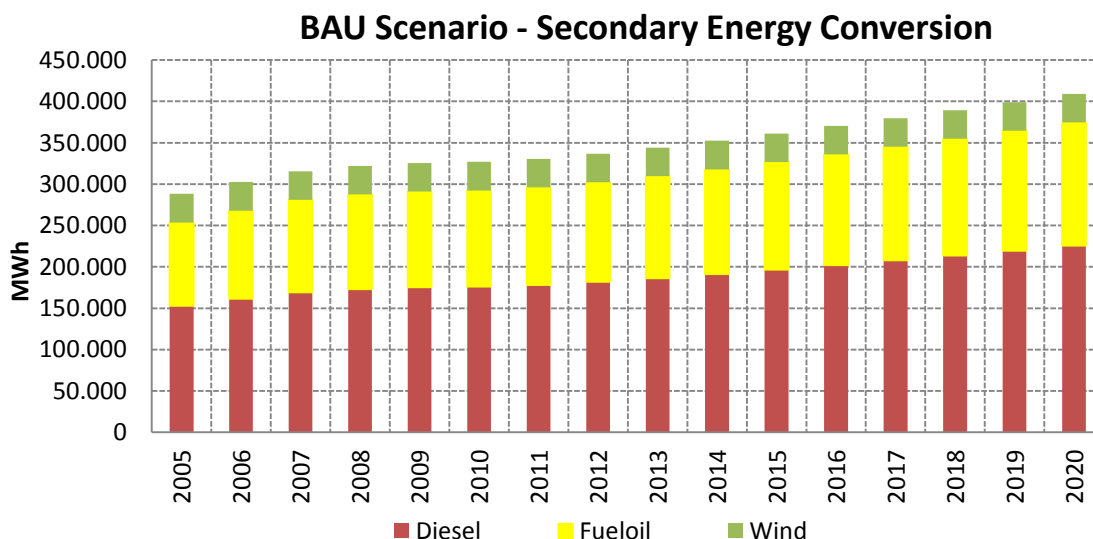
Διάγραμμα 3.24. BAU σενάριο – Δευτερογενής μετατροπή ενέργειας για παραγωγή ηλεκτρισμού
